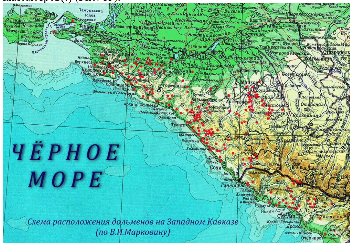
Рис. 15. Схема расположения дольменов на Западном Кавказе.
